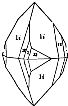
Schlackenwald.
